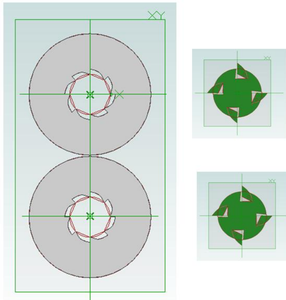
Ilustração 4 – Rodas dentadas com os socalcos e detalhe dos dentes dos veios/Inner diameter of the main gears and the shaft locking detail.
